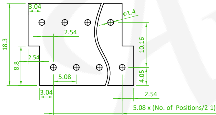
P.C.B. LAYOUT
