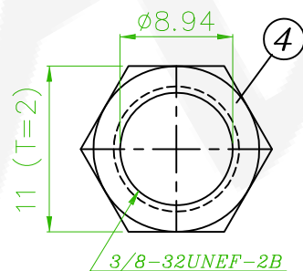
CLAMP NUT
