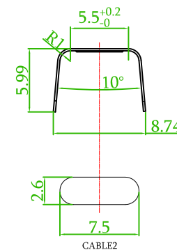
TYPE2(OD7.5*2.6)
