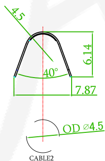
TYPE-2(ODØ4.5)
