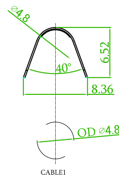
TYPE1(ODØ4.8)
