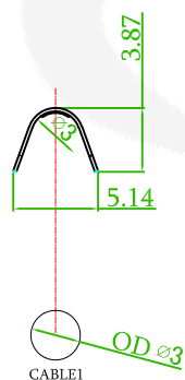
TYPE-1(ODØ3.0)
