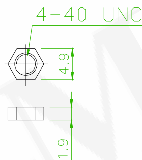
(D)NUT
