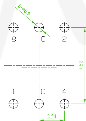
P. C. B. LAYOUT
