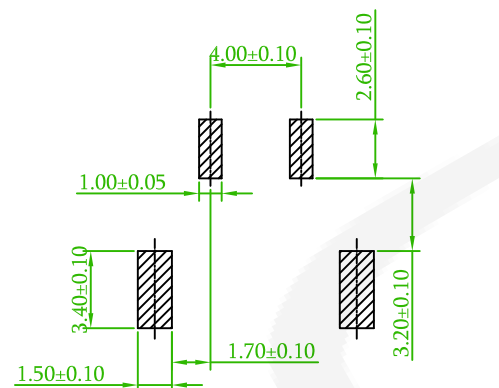
P.C.B LAYOUT
