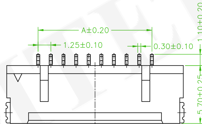
04P~30P
