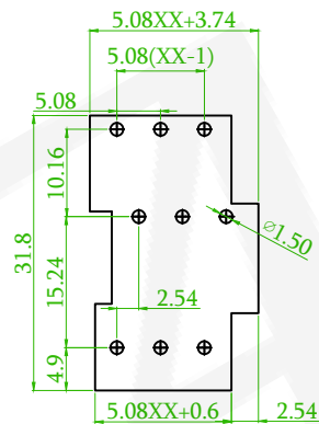
P.C.B. LAYOUT
