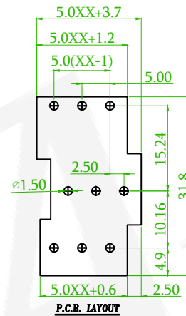
P.C.B. LAYOUT
