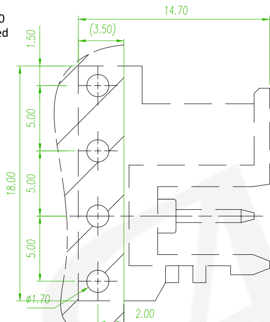
P.C.B. LAYOUT
