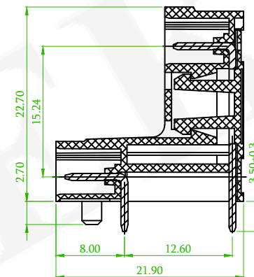
SECTION:P-P
