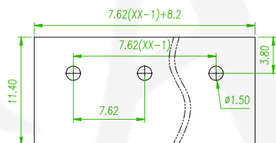
P.C.B. LAYOUT
