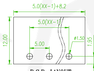
P.C.B. LAYOUT
