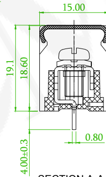
SECTION A-A
