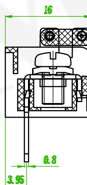
SECTION A-A
