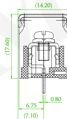
SECTION A-A
