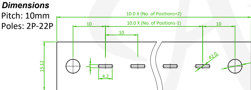
P.C.B. LAYOUT
