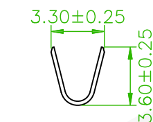
SEC:A-A
