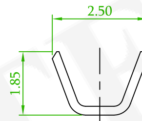
SEC:A-A
