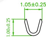
SEC:B-B
