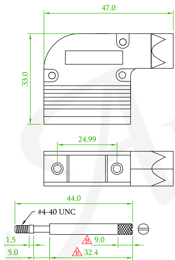
Long Bolt
