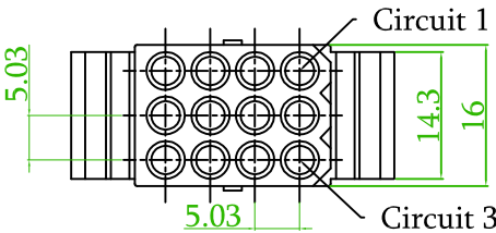
3X4 PIN
