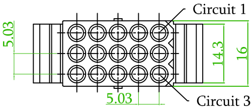
3X5 PIN
