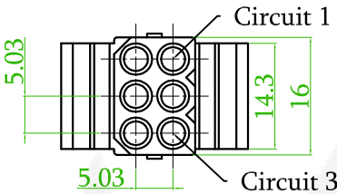
3X2 PIN
