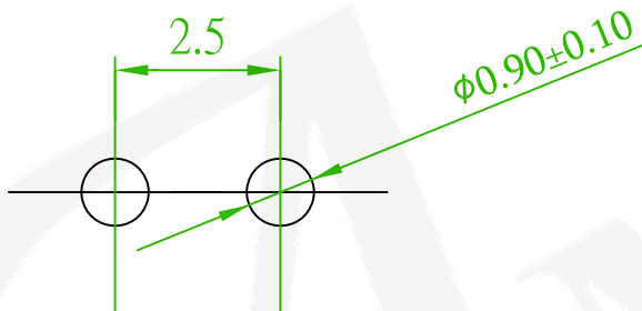
HOLE IN P.C.B
