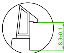
Long Ejector
